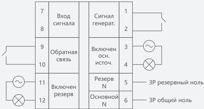
Примечание: внешний дополнительный источник Схема подключения контроллера типа В
