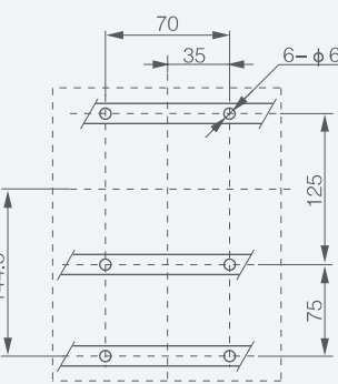
4P: монтаж на направляющие
