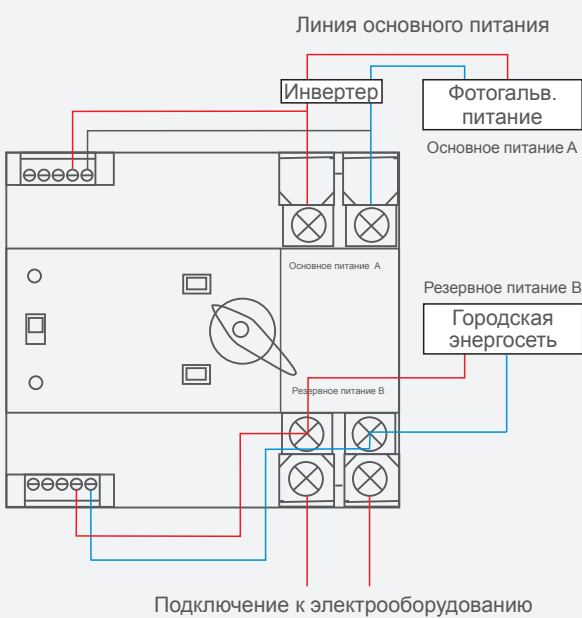
Специальный режим подключения фотогальванического инвертора YCQ4R Рис.6
