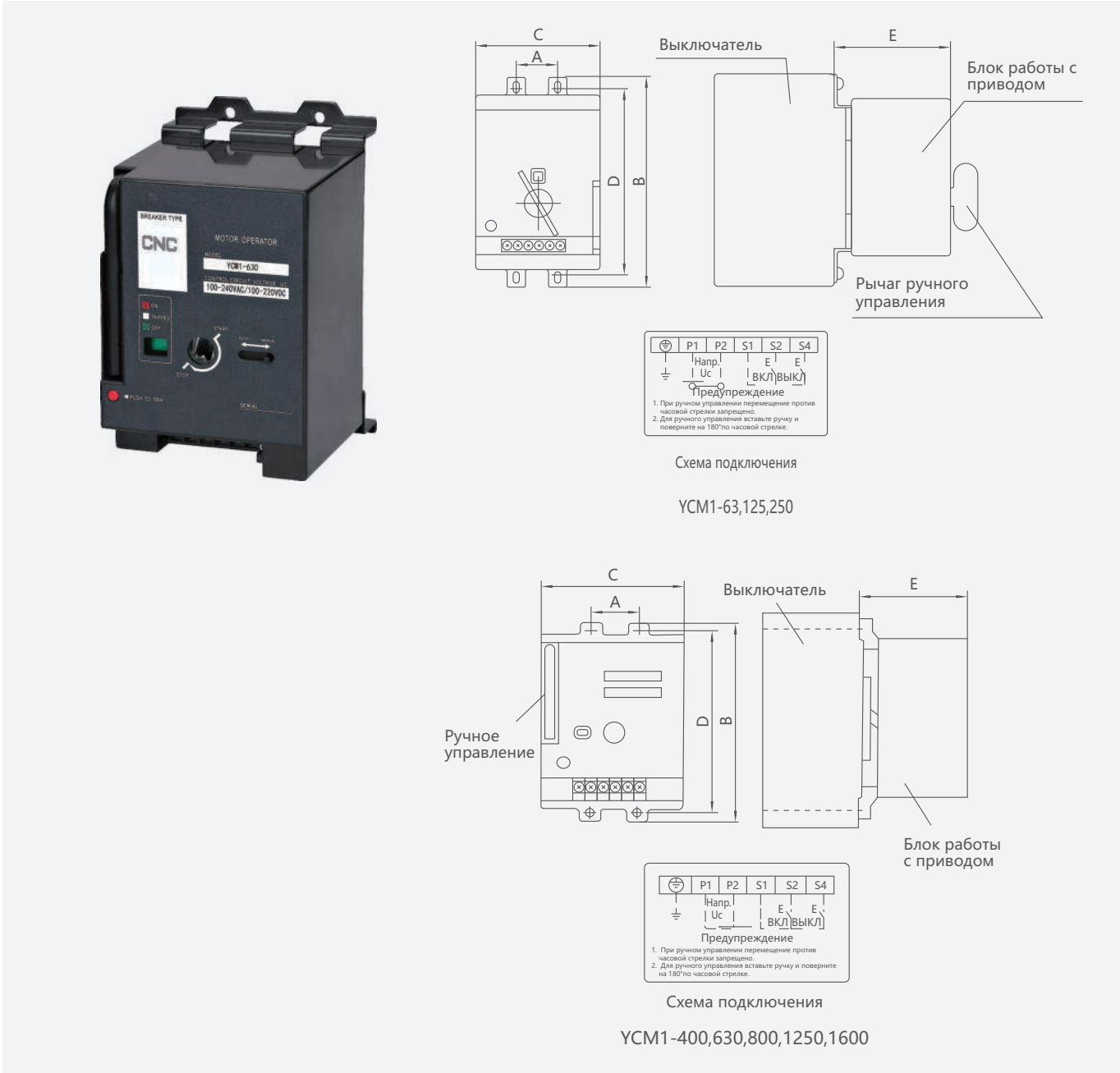
Габаритные и монтажные размеры (мм)
