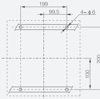
3P: монтаж на направляющие
