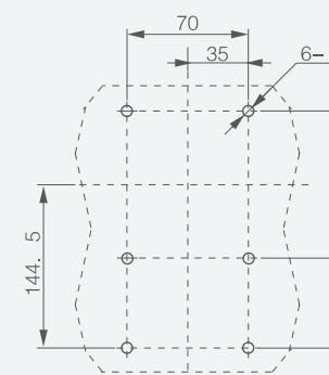
4P: монтаж на панель
